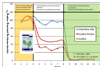
Tests en chambre environnementale mettant en évidence l'adsorption irréversible du formaldéhyde
