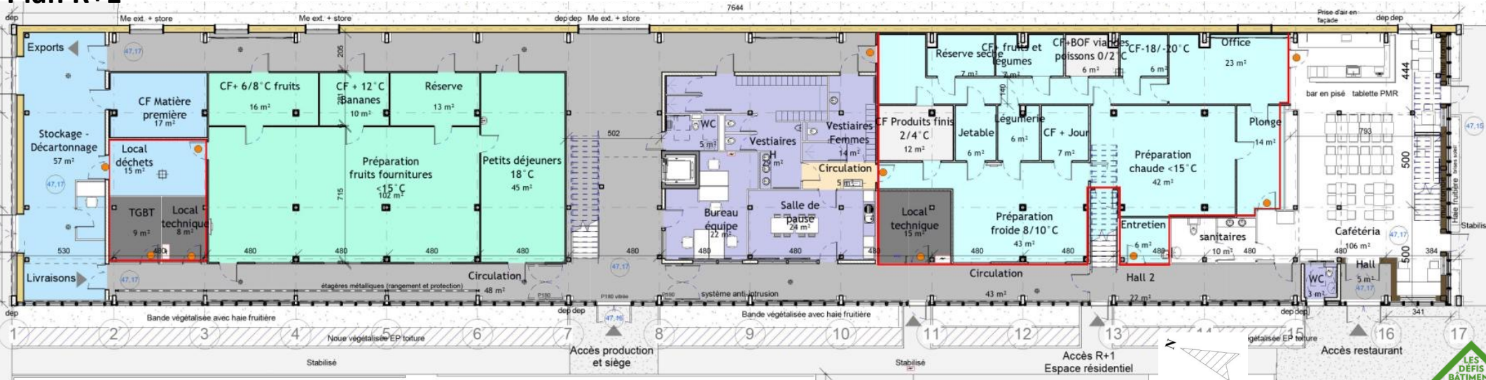
Plan rez-de-chaussée
